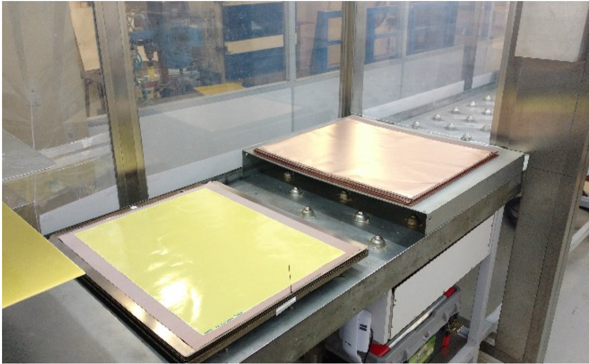
Figura 3 – Montagem do Stackup 2
